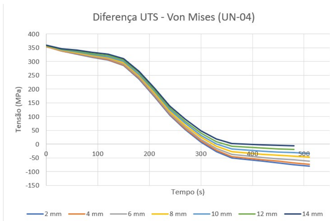
Figura 4.29: Otimização do diâmetro do FO - UN-03 - Diferença mínima entre a tensão UTS e Von Mises.
