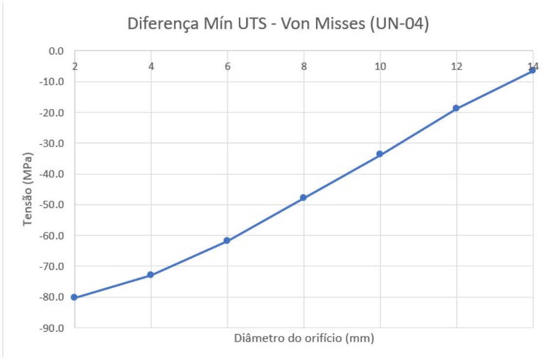
Figura 4.31: Otimização do diâmetro do FO - UN-04 - Diferença mínima entre a tensão UTS e Von Mises.
