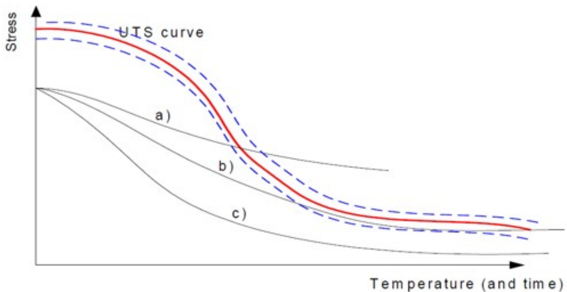
Figura 3.5: Curvas de tensão máxima admissível (UTS) e tensão aplicada (Von Mises) (HEKKELSTRAND e SKULSTAD, 2004).
