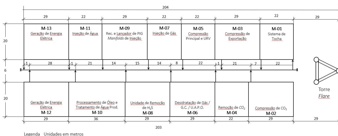
Figura 3.1: Arranjo das tubulações - vista superior no FPSO.
