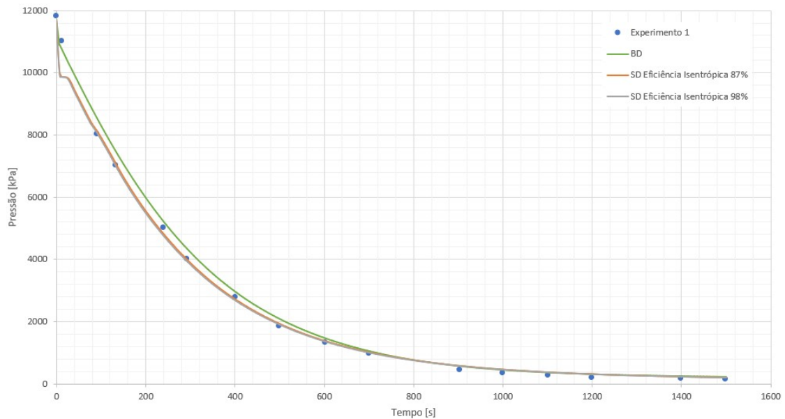
Figura 4.11: Experimento 1 - Pressão (SD vs Experimental vs BD).
