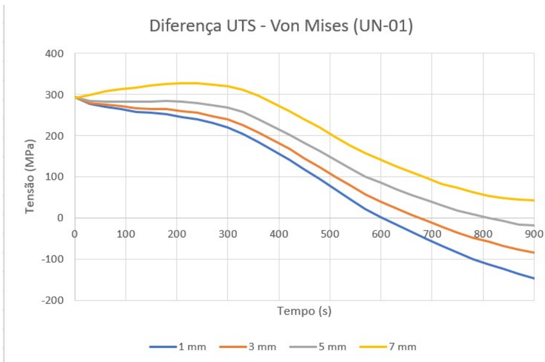
Figura 4.24: Otimização do diâmetro do FO - UN-01 - Diferença entre a tensão UTS e Von Mises ao longo da depressurização.
