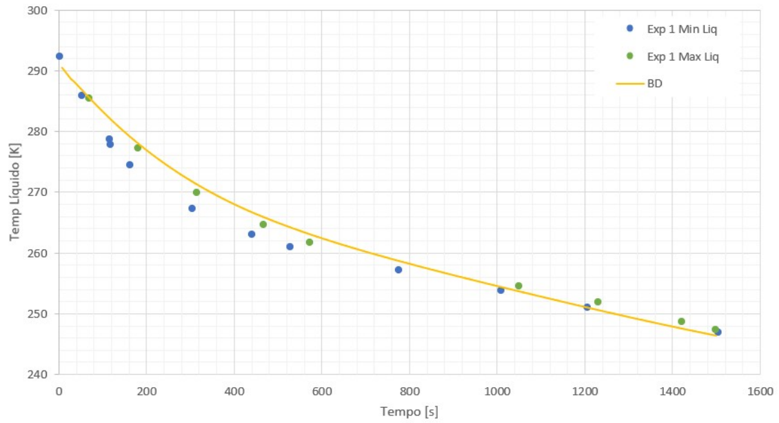
Figura 4.2: Experimento 1 - BD - Temperatura da fase líquida.
