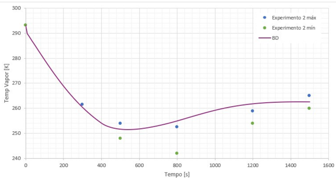
Figura 4.8: Experimento 2 - BD - Temperatura da fase vapor.
