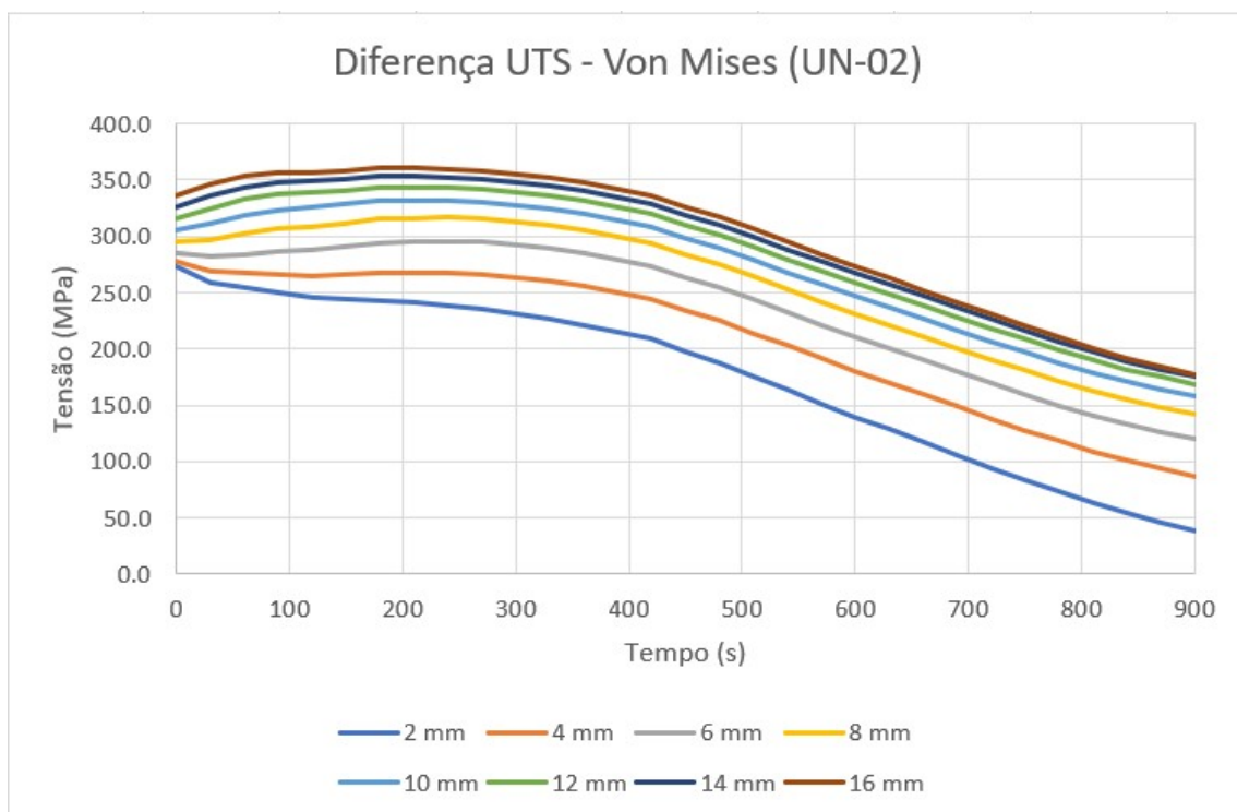
Figura 4.26: Otimização do diâmetro do FO - UN-02 - Diferença entre a tensão UTS e Von Mises ao longo da depressurização.
