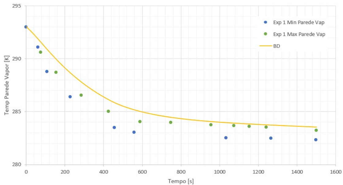
Figura 4.5: Experimento 1 - BD - Temperatura da parede metálica em contato com a fase vapor.
