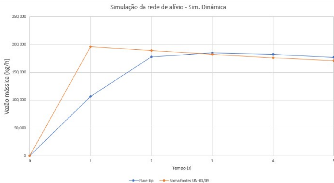
Figura 4.22: Simulação da rede de alívio - SD - 0-5 s.
