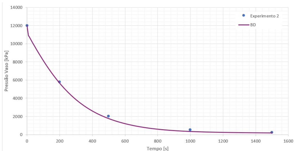
Figura 4.6: Experimento 02 - BLOWDOWN - Pressão.
