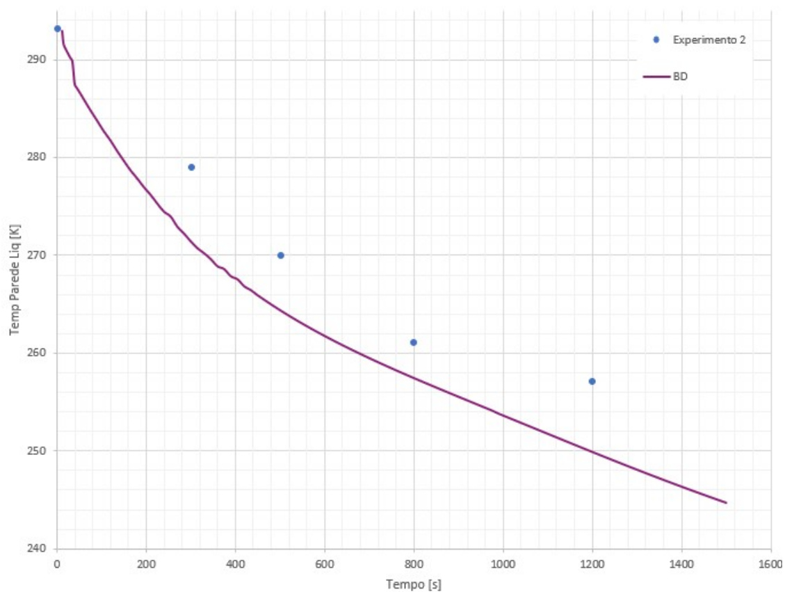
Figura 4.9: Experimento 2 - BD - Temperatura da parede metálica em contato com a fase líquida.
