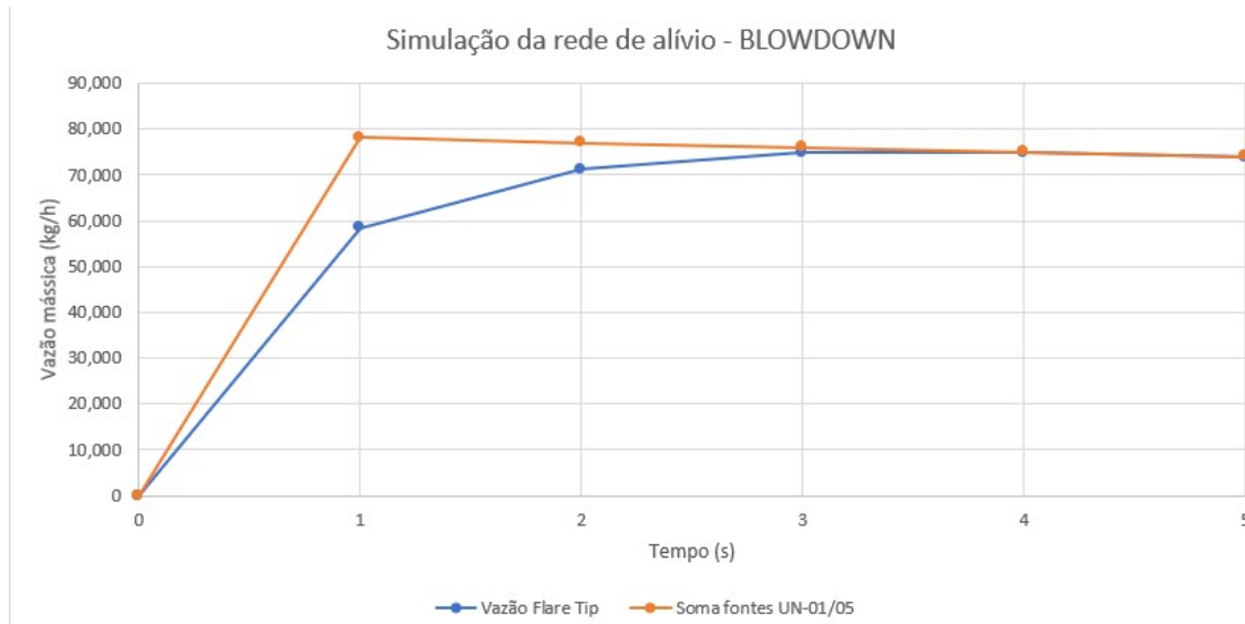
Figura 4.23: BD - Resultado simulação considerando influência dos volumes das tubulações no pico de vazão no flare tip .
