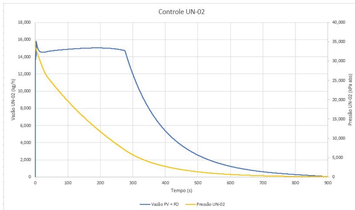
Figura 4.35: Controle da vazão de despressurização - UN-02 - Pressão e Vazão total despressurizada para a UN-02.
