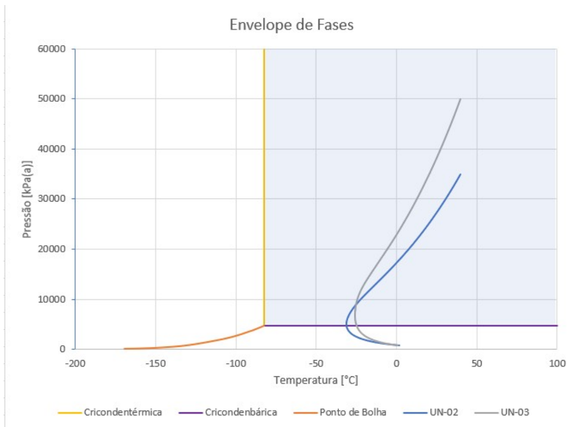
Figura 4.21: Envelope de fases para metano - Caminho de despressurização das fontes UN-02/03 e região supercrítica.
