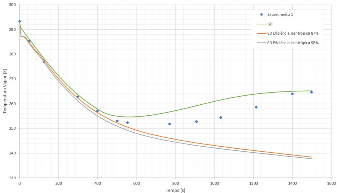
Figura 4.13: Experimento 1 - Temperatura da fase vapor (SD vs Experimental vs BD).
