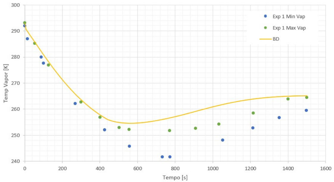
Figura 4.3: Experimento 1 - BD - Temperatura da fase vapor.
