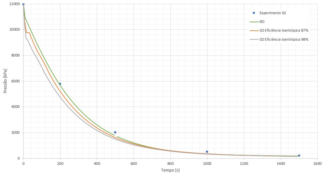
Figura 4.16: Experimento 2 - Pressão (SD vs Experimental vs BD).
