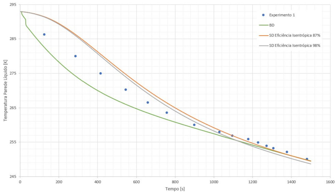
Figura 4.14: Experimento 1 - Temperatura da parede metálica em contato com a fase líquida (SD vs Experimental vs BD).
