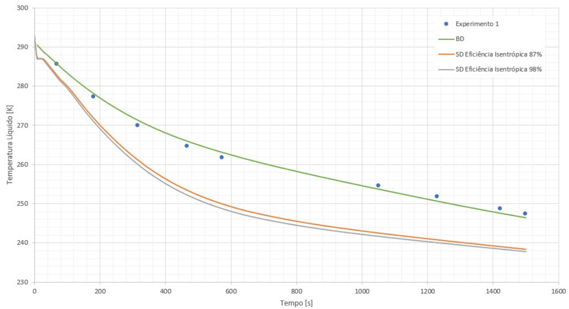
Figura 4.12: Experimento 1 - Temperatura da fase líquida (SD vs Experimental vs BD).
