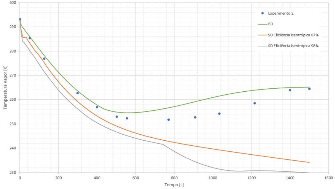
Figura 4.18: Experimento 2 - Temperatura da fase vapor (SD vs Experimental vs BD).
