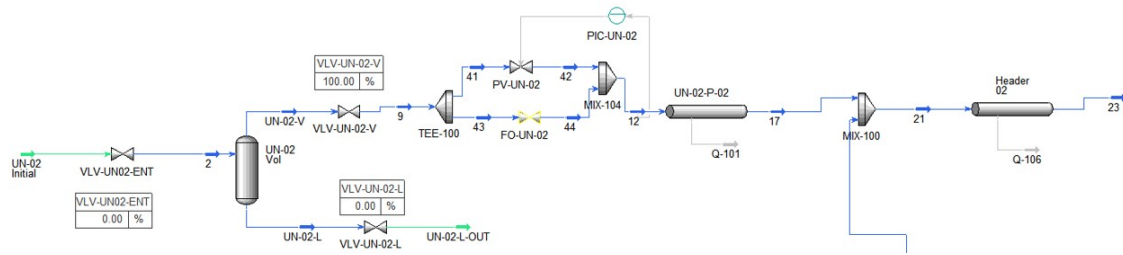
Figura 3.6: Arranjo do controle proposto.
