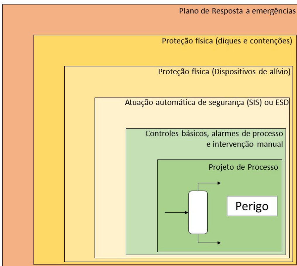
Figura 1.1: Camadas de proteção em uma unidade industrial (WILLEY, 2014).
