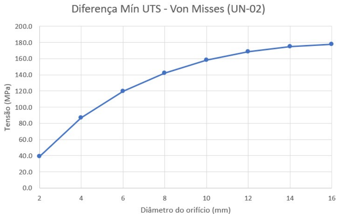
Figura 4.26: Otimização do diâmetro do FO - UN-02 - Diferença entre a tensão UTS e Von Mises ao longo da depressurização.
