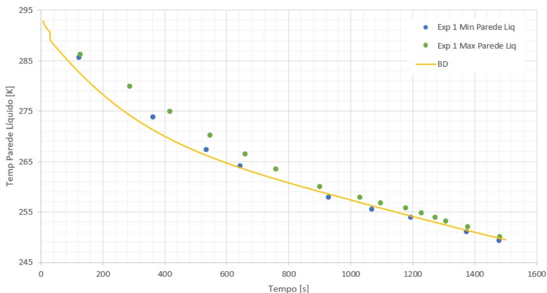
Figura 4.4: Experimento 1 - BD - Temperatura da parede metálica em contato com a fase líquida.
