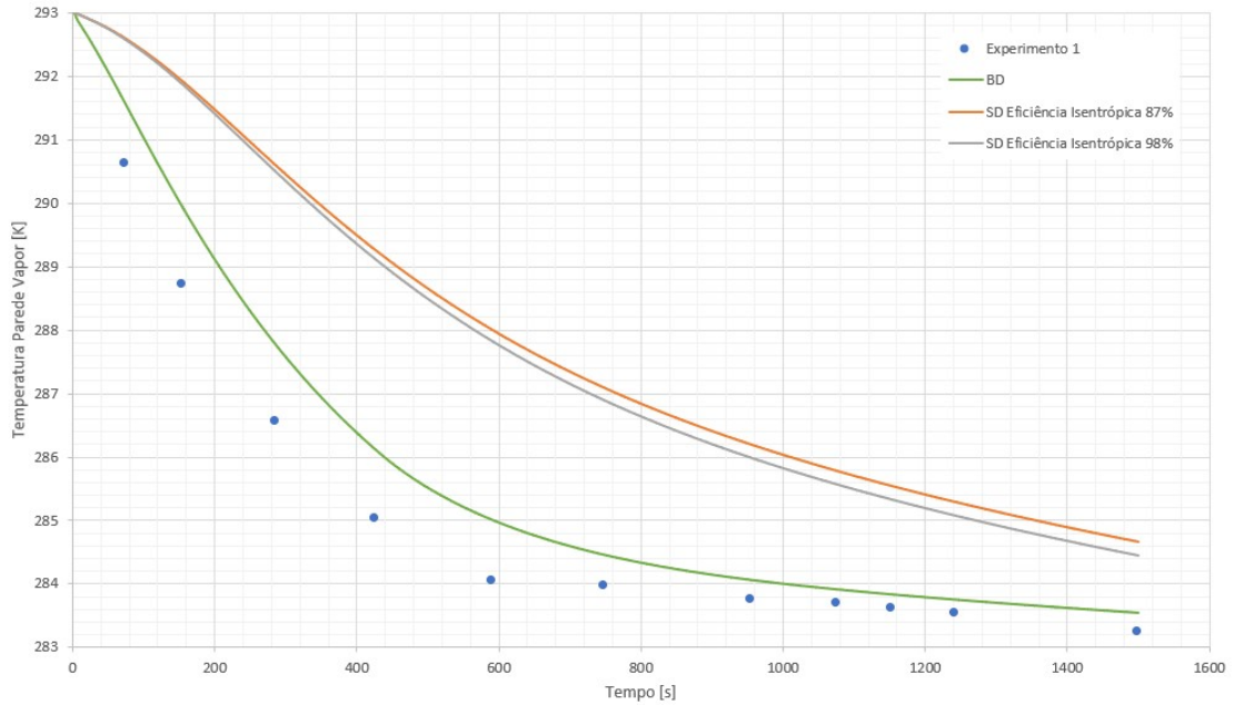
Figura 4.15: Experimento 1 - Temperatura da parede metálica em contato com a fase vapor (SD vs Experimental vs BD).
